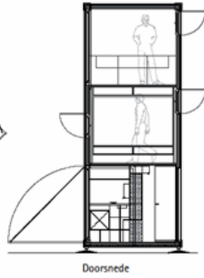
Doorsnede
